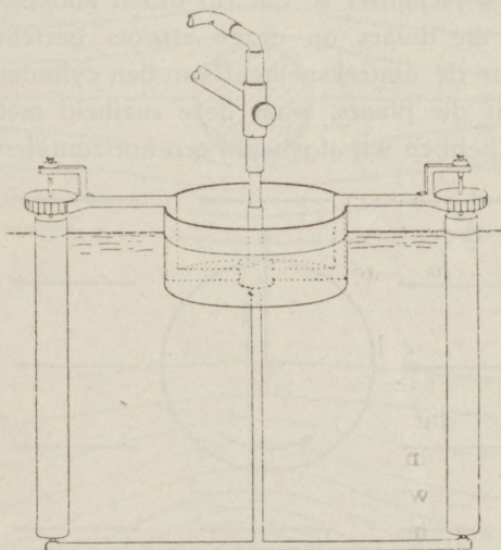
Fig. 2. Aantrekking of afstooting tusschen roteerende cylinders. De figuur laat de drijvende opstelling zien van de roteerende cylinders die bewegelijk zijn. Nog zoo'n cylinder kan met een handvat in de hand genomen of in een statief vastgeklemd worden. De rotatie wordt door aanblazen, tegen de schoep-raadjes bovenaan, onderhouden.
